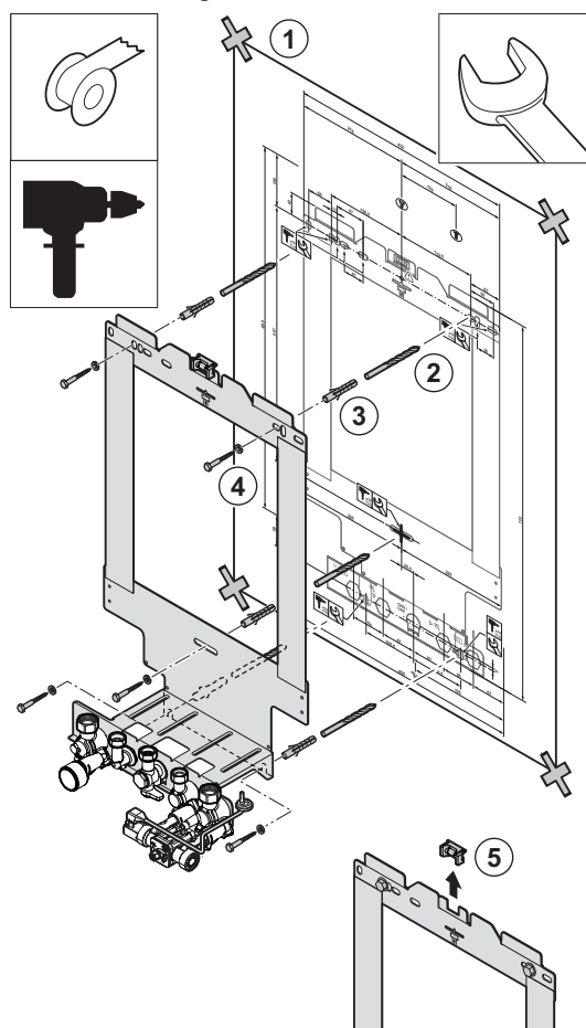
Afb.10 Montageframe installeren
