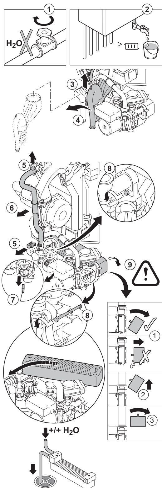
Afb.105 Reiniging platenwarmtewisselaar
