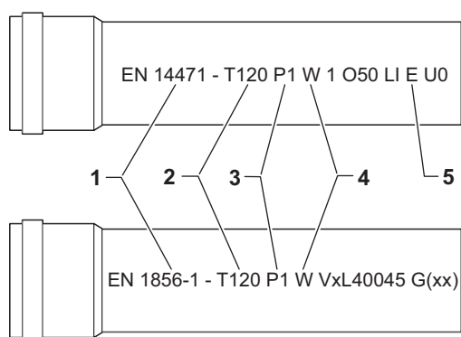
Afb.19 Voorbeelden tekenreeks
