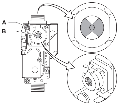
Afb.72 Afstelschroef A
