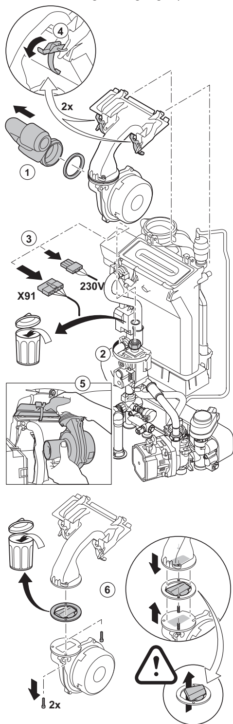
Afb.109 Vervangen terugslagklep
