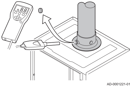
Afb.66 Rookgasmeetpunt
