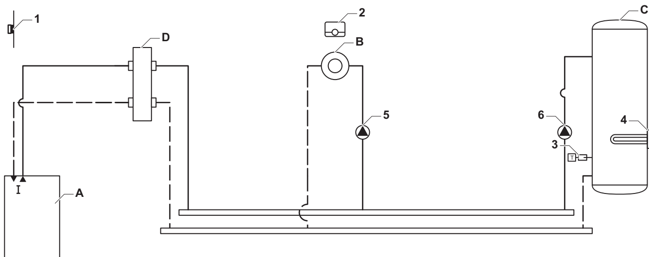
Afb.51 1 ketel + 1 LLH + 1 directe zone + warmwaterzone met elektrisch verwarmingselement
