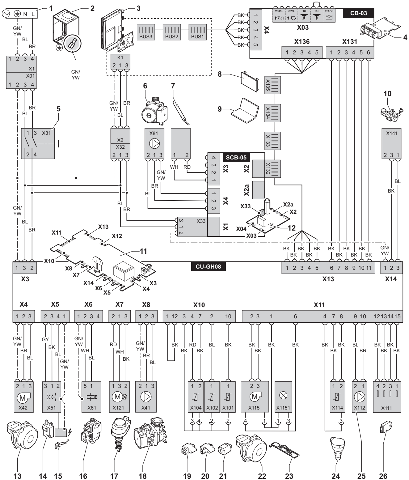
Afb.2 Elektrisch schema
