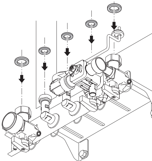
Afb.12 Plaatsen pakkingringen
