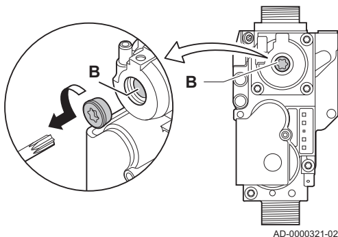
Afb.70 Positie afstelschroef B
