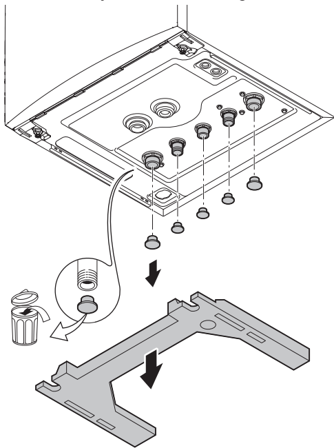
Afb.11 Verwijderen bescherming ketel
