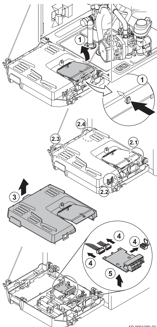
Afb.111 Toegang tot de aansluitconnectoren
