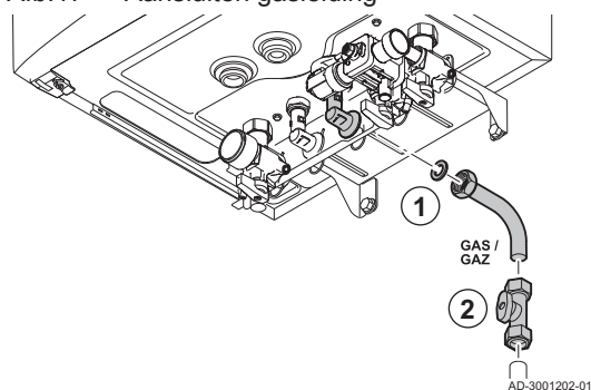
Afb.17 Aansluiten gasleiding
