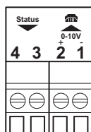
Afb.43 Ingangs-/uitgangsconnector
