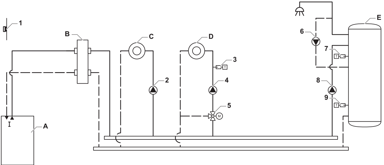
Afb.53 1 ketel + 1 LLH + 1 directe zone + mengzone + warmwaterzone
