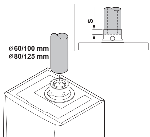
Afb.27 Aansluiten rookgasafvoer en luchttoevoer
