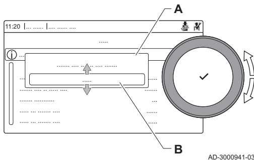
Afb.67 Vollasttest
