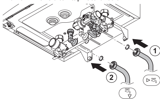
Afb.15 Aansluiten tapwatercircuit
