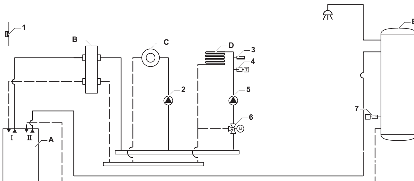
Afb.52 1 ketel + 1 LLH + 1 directe zone + mengzone + warmwaterzone
