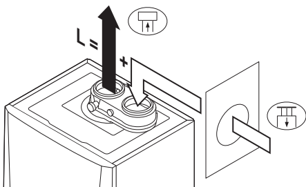
Afb.25 Verschillende drukgebieden
