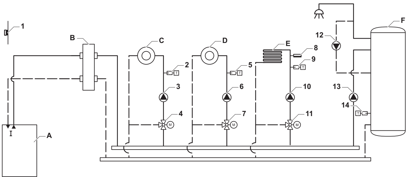
Afb.55 1 ketel + 1 LLH + 3 meng zones + warmwaterzone
