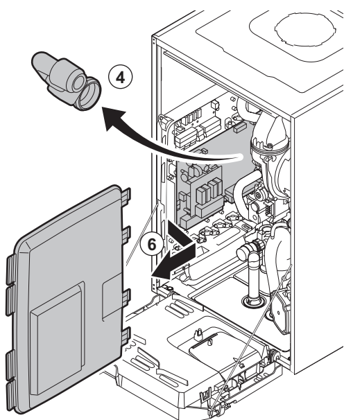
Afb.37 Toegang tot de besturingsprint
