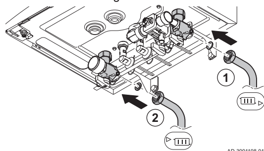
Afb.14 Verwarmingscircuit aansluiten
