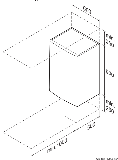
Afb.8 Montageruimte
