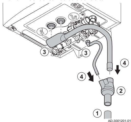
Afb.16 Condensafvoerbuis aansluiten
