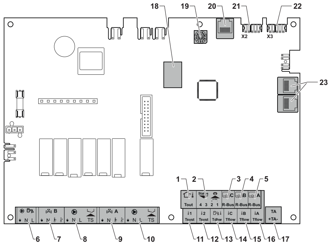
Afb.38 SCB-10-printplaat
