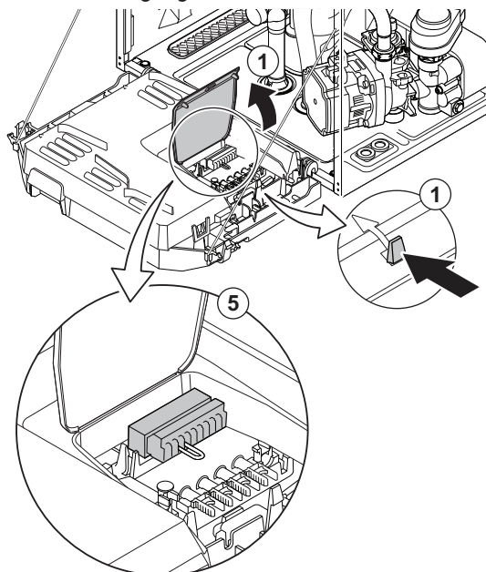
Afb.28 Toegang tot de aansluitconnectoren
