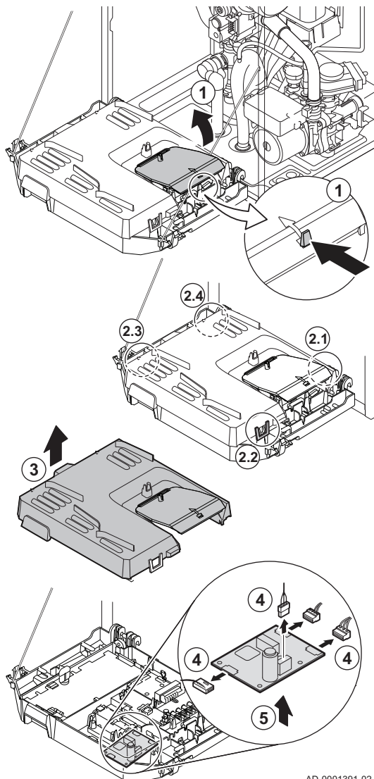
Afb.112 Toegang tot de aansluitconnectoren
