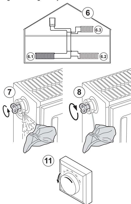
Fig.18 Purge du système
