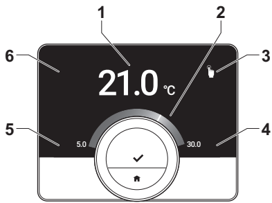
Afb.10 Display van de thermostaat
